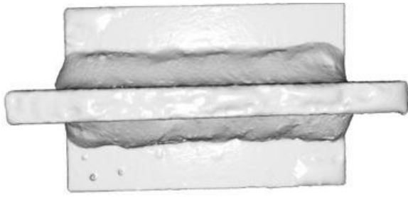
2. ábra Hibátlan és hibával rendelkező pontfelhő
