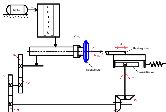
10. ábra. Hátraesztérge gép elvi felépítése
